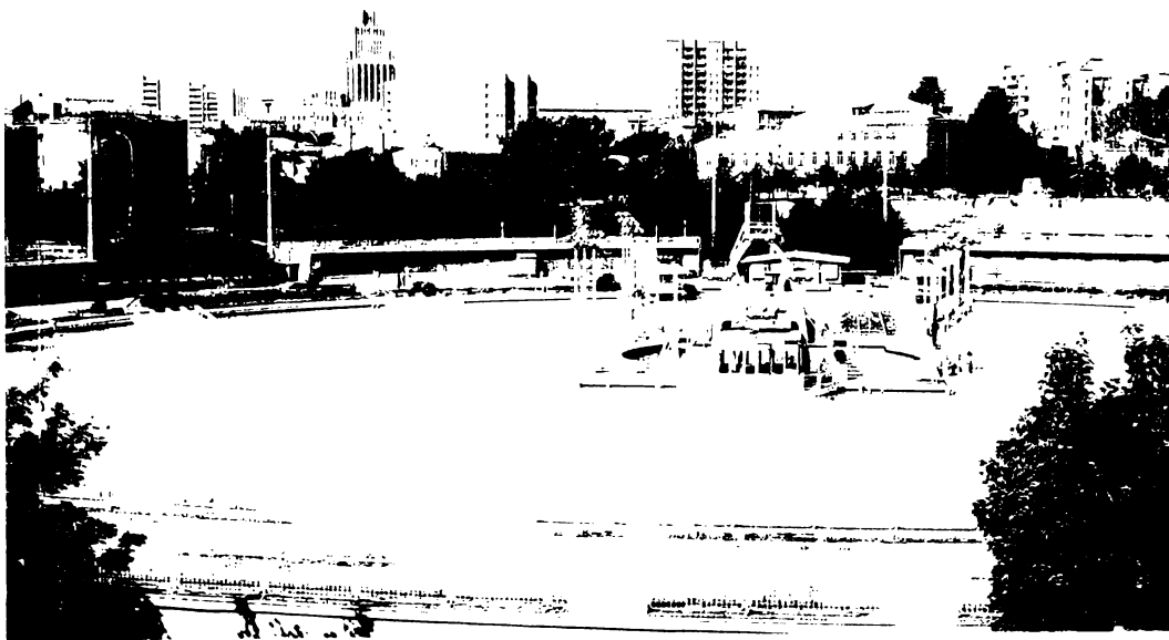
Бассейн «Москва»
